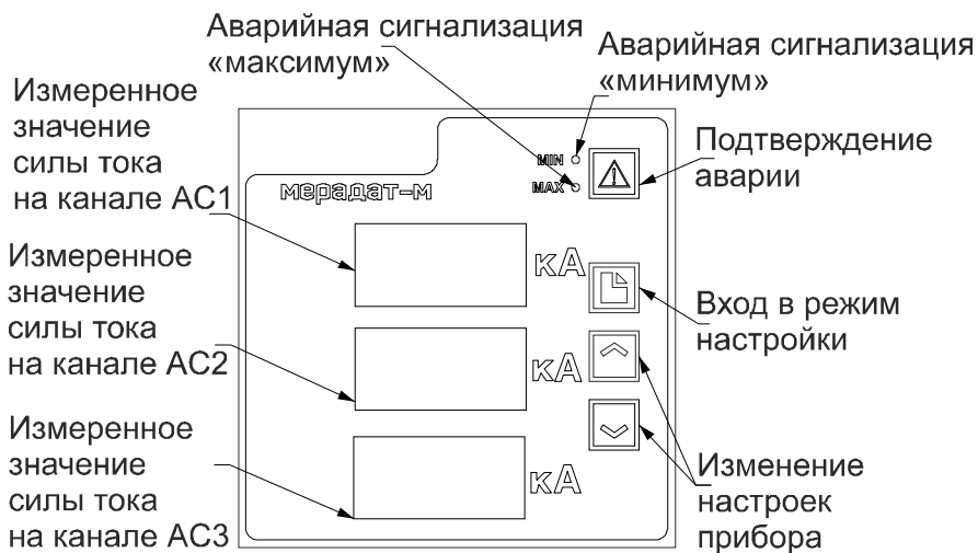
Рисунок 3 - Вид передней панели прибора, модель Мерадат-М3А
